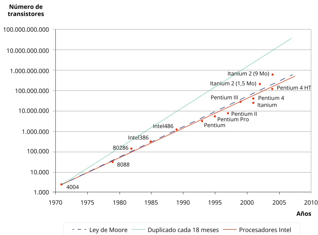
Gráfica 1. Desarrollo tecnológico (número de transistores por años).
